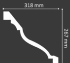
▲ PU-KRP-019
